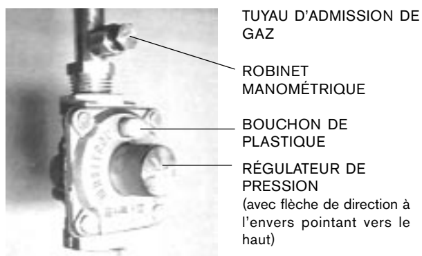
Fig. 5 - Installation régulateur de pression du gaz
