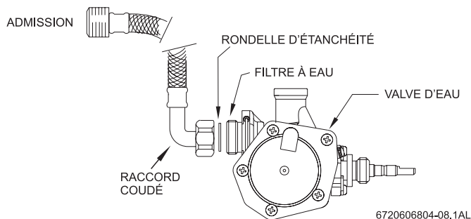
Fig. 6 - Valve d'eau et manchon de raccordement (vue d'en haut)
