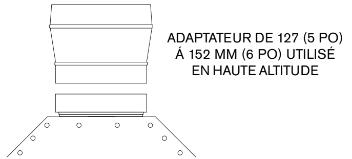
Fig. 4 - Adaptateur du conduit d'évacuation pour un chauffe-eau installé en haute altitude
