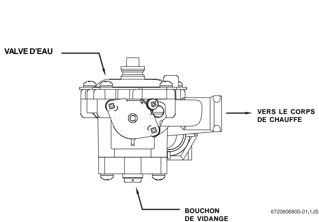
Fig. 1 - Bouchon de vidange du chauffe-eau
