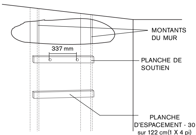
Fig. 2 - Montage du chauffe-eau
