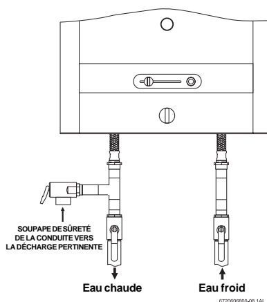
Fig. 7 - Soupape de sûreté
