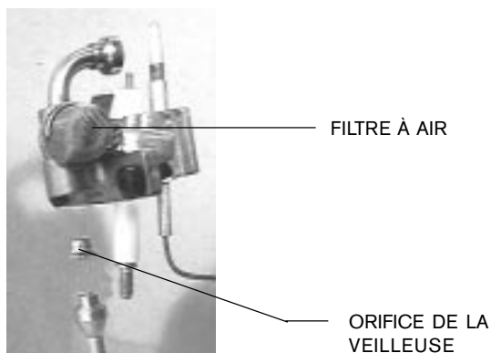
Fig. 11 - Brûleur, filtre à air et orifice de la veilleuse
