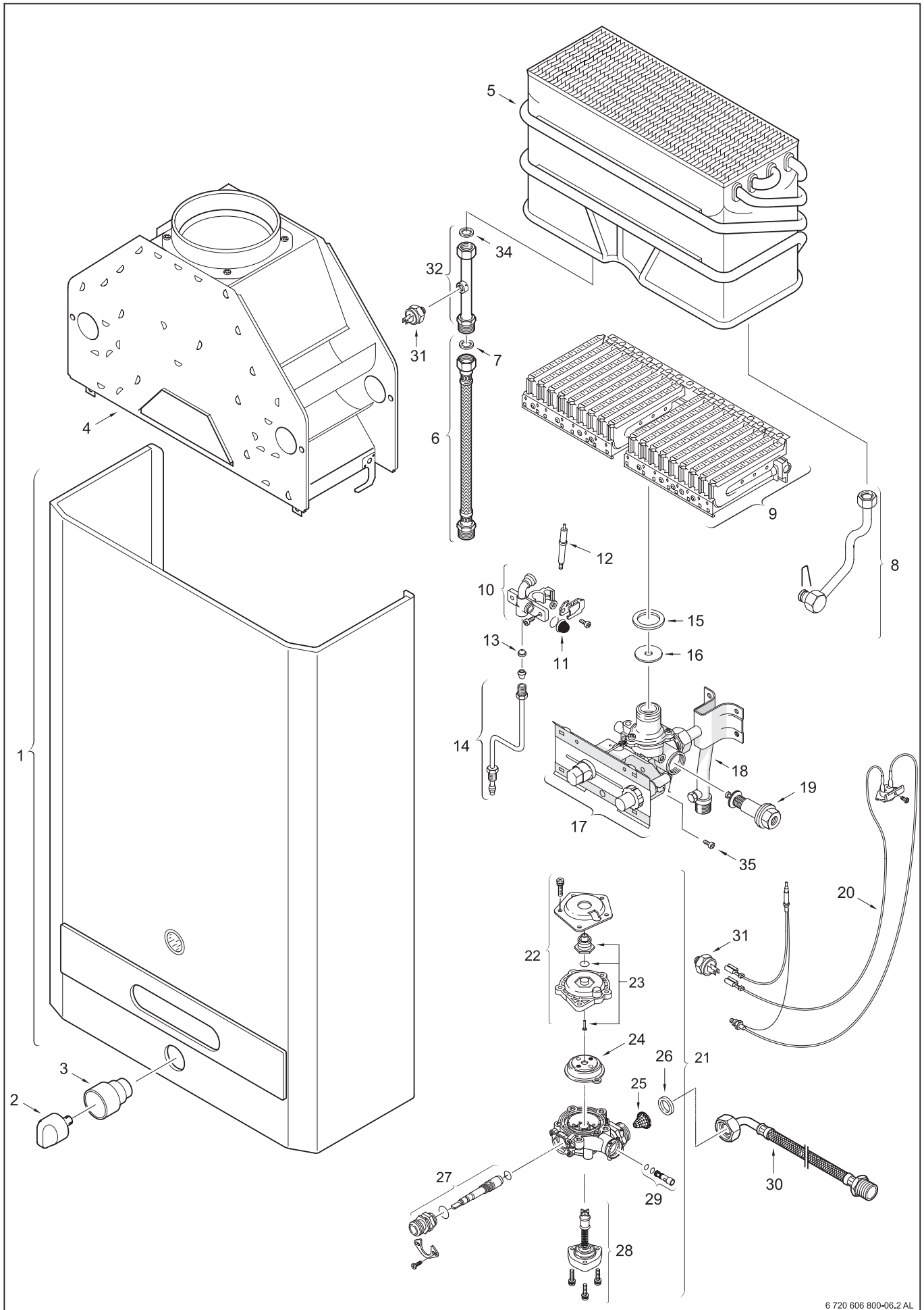
Fig. 13 - Diagramme des composants intérieurs et liste des pièces de l'aquastar 125B
