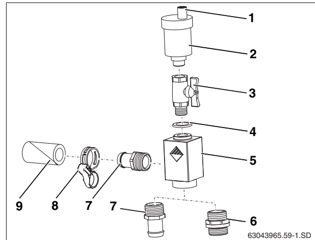
Fig. 59 Universal air vent set
